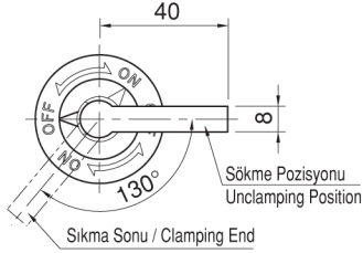
Ürün Nr. 1489 Tek Dokunuş Bağlama • Siyah Kaplama
