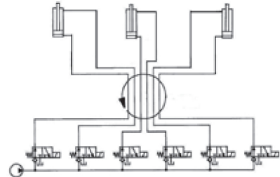
Hidrolik Devre Şeması Hydraulic Circuit Diagram
