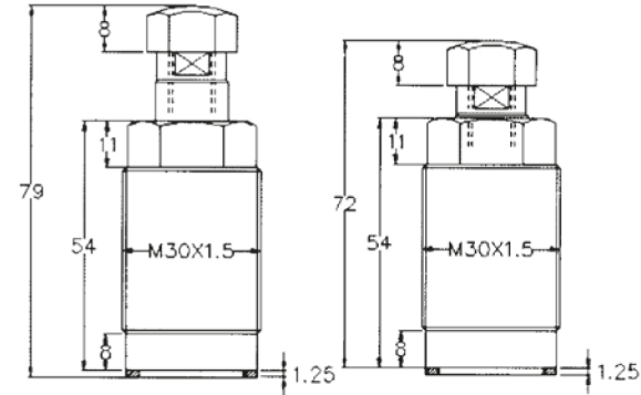
Ürün Nr. 1056 Hidrolik İş Parçası Desteği
